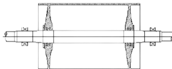
Fig 11 – Fixação de tambores para transportadores de correia
