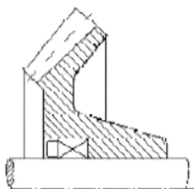
Fig 10 – Fixação de engrenagens
