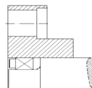
Fig 8 – Fixação de embreagens e acoplamentos
